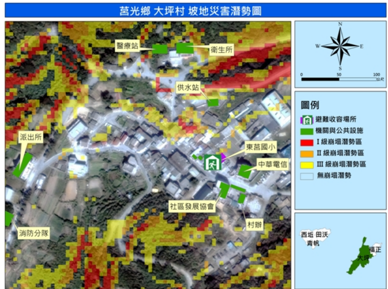
圖2-42 大坪村坡地災害潛勢圖
